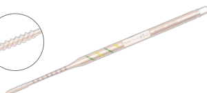
93320602-93024002 双线丝锥 Tap, Φ5.0 曾用编码 93100201
