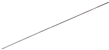
91123201 螺纹导针 Threaded Guide Pin, \Phi 3.2 \times 400\text{mm}
