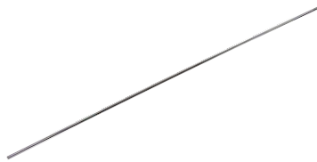
91123201 螺纹导针 Threaded Guide Pin, \Phi 3.2 \times 400\text{mm}
